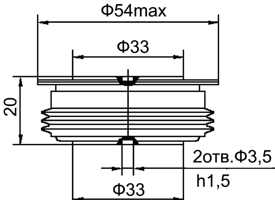
Рис. 11. Габаритные и установочные размеры
