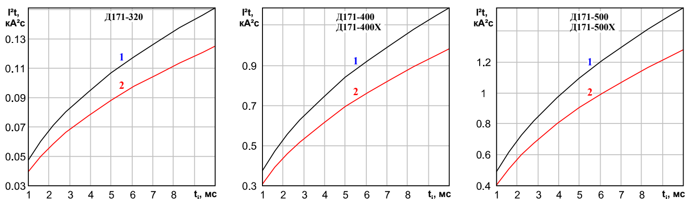
Рисунок 5: Зависимость защитного показателя I^2t от длительности импульса тока t_p при исходной температуре структуры T_j=25^\circ\text{C} (1) и максимально допустимой температуре перехода T_{jm} (2).
