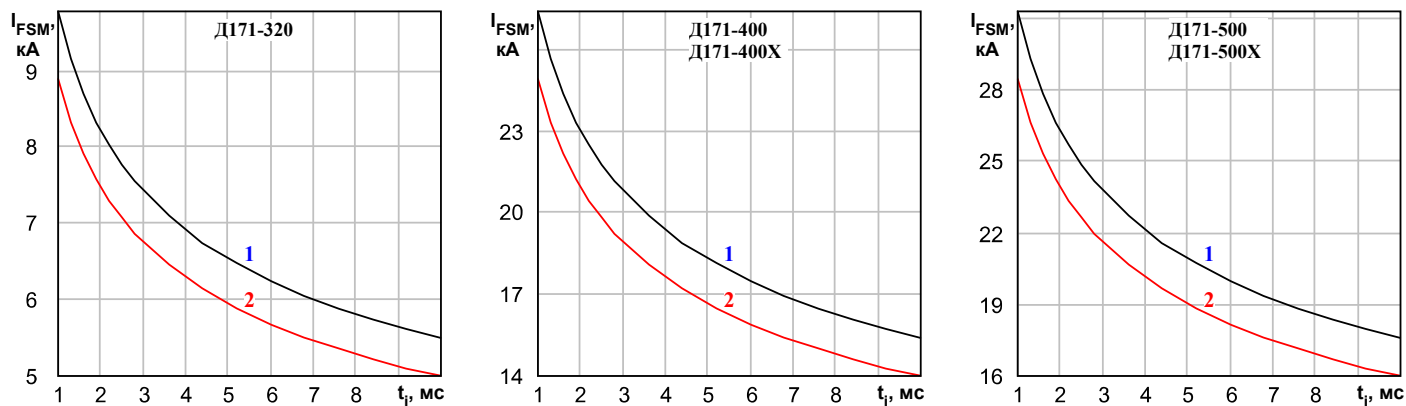
Рисунок 4: Зависимость допустимой амплитуды ударного прямого тока I_{FSM} от длительности импульса тока t_p при исходной температуре структуры T_j=25^\circ\text{C} (1) и максимально допустимой температуре перехода T_{jm} (2).
