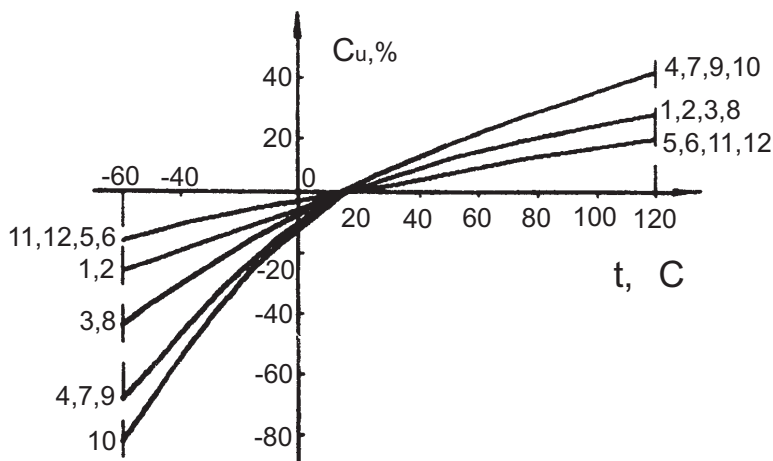
Изменение ёмкости от температуры
