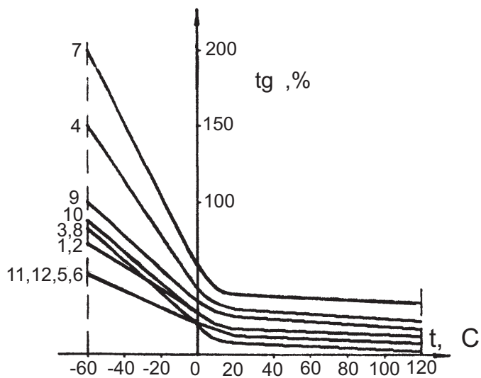
Изменение тангенса угла потерь от температуры
